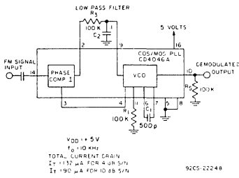
Fig. 10— FM demodulator.
