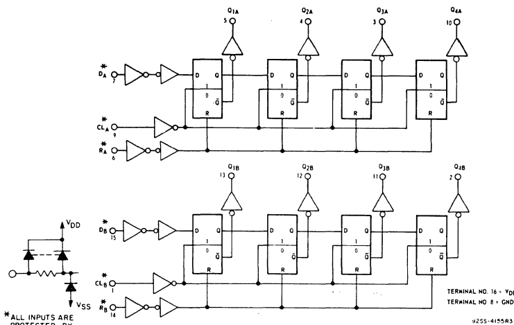
Fig. 6 - Logic diagram.
