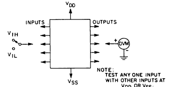
Fig. 16 - Input voltage test circuit.
