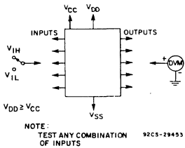
Fig. 14 - Input voltage.
