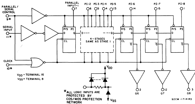
Fig. 5 - Logic diagram.
