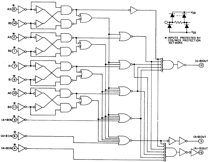
Fig. 4 - Logic diagram.
