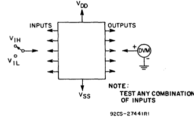
Fig. 16 - Input voltage.
