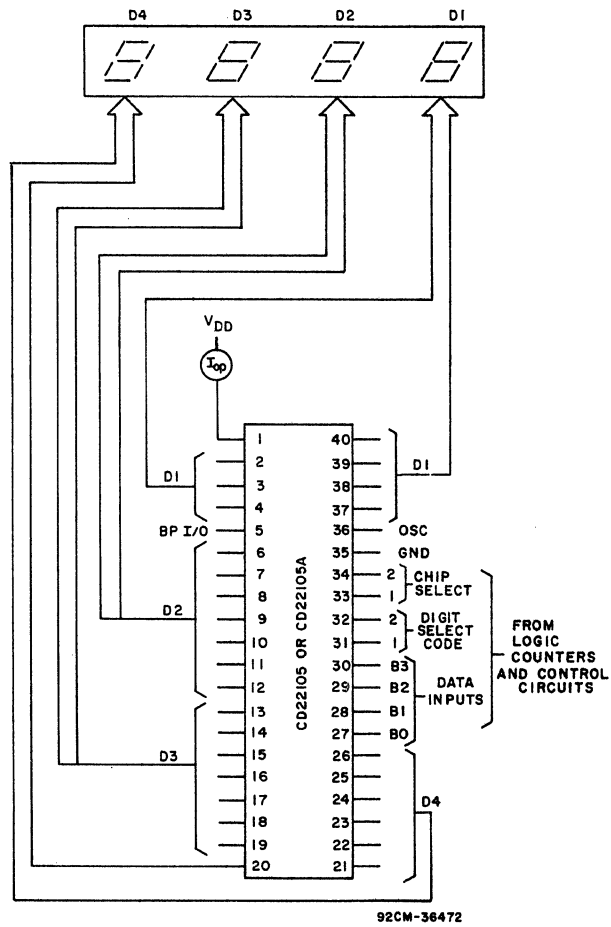
Fig. 5 - Test circuit.
