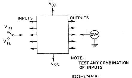
Fig. 14 - Input voltage.
