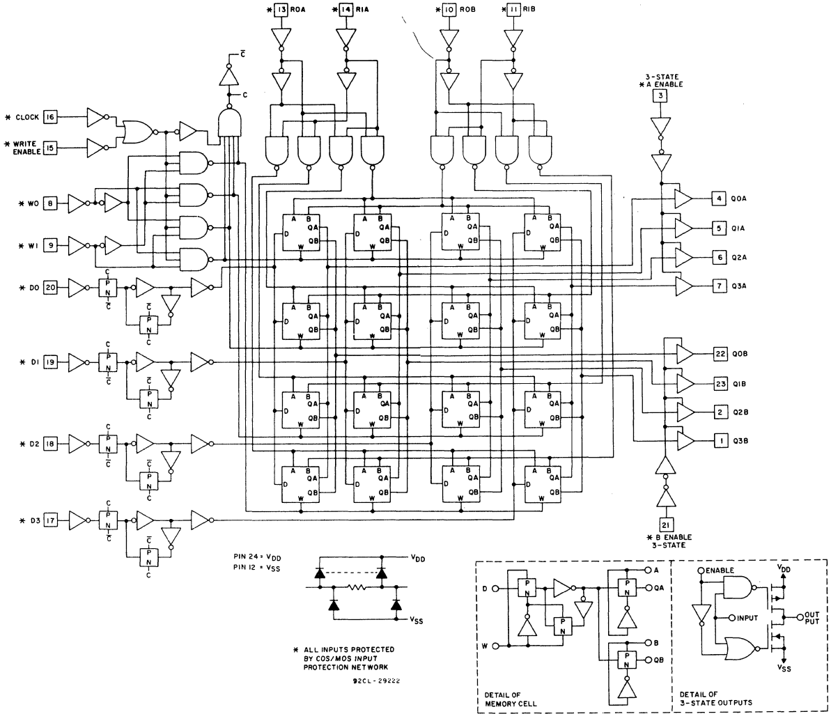
Fig. 2 - Logic diagram.
