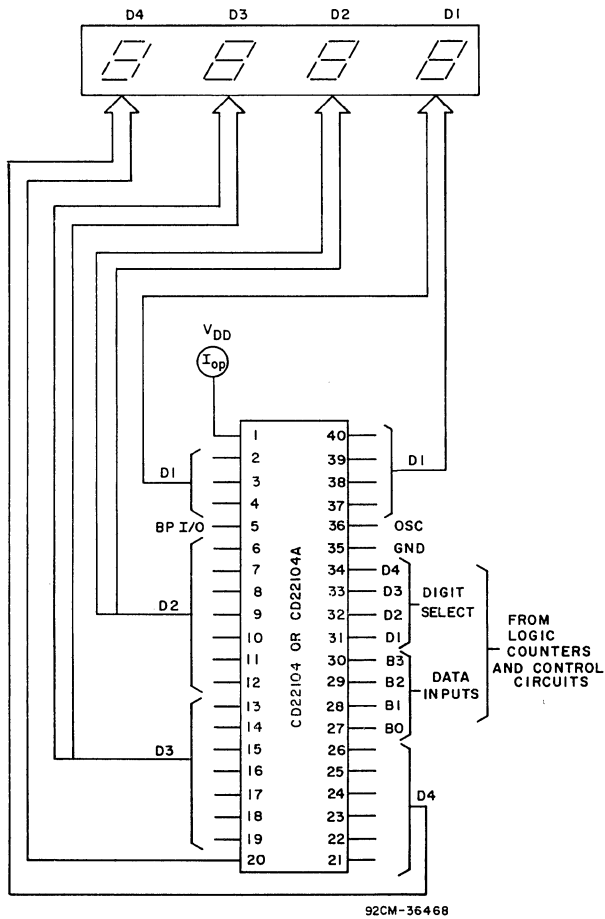
Fig. 5 - Test circuit.
