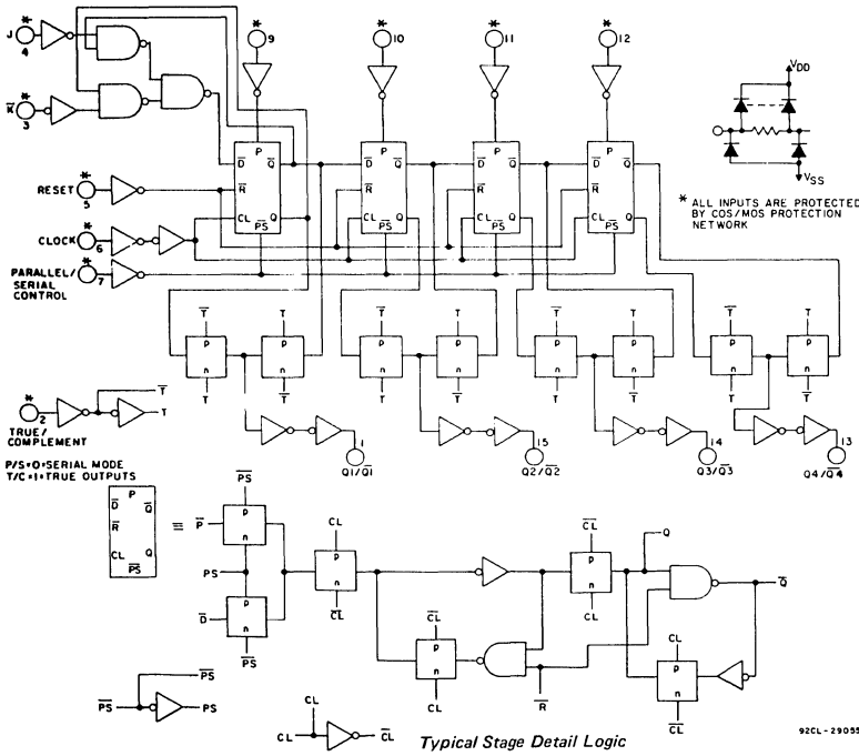
Fig. 4 - Logic diagram.
