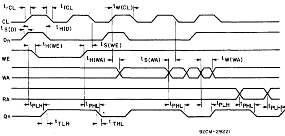
Fig. 4— Timing diagram.
