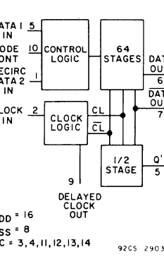
92CS-29039 64-Stage Static Shift Register CD4031A (Page 543) CD4031B (Page 149)
