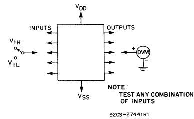
Fig. 25—Input-voltage test circuit.
