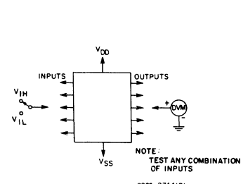
Fig. 13 - Input voltage test circuit.
