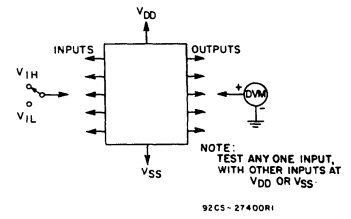
Fig. 11 - Input voltage.
