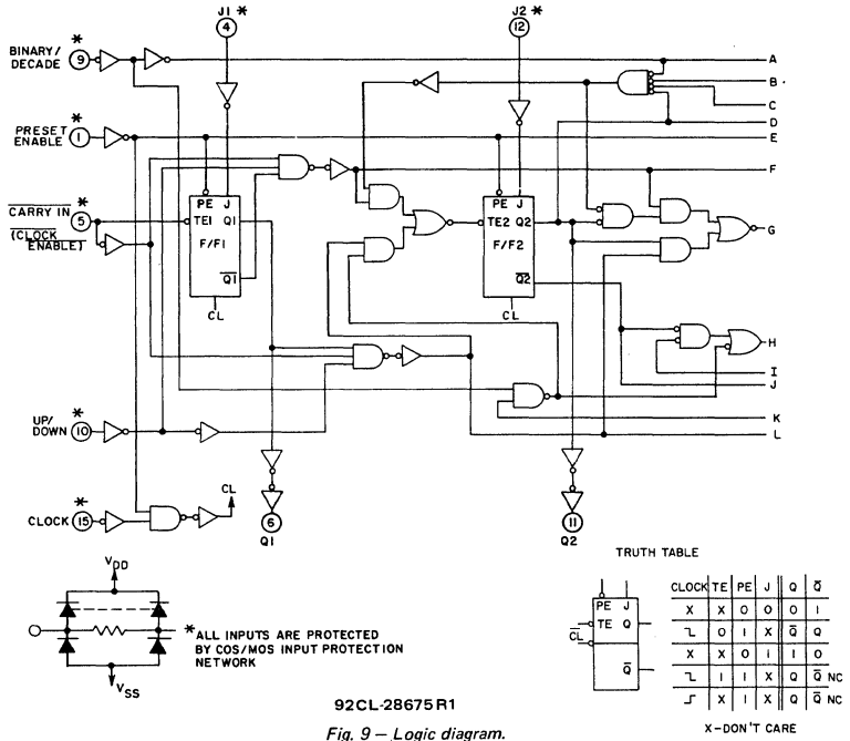
Fig. 9 - Logic diagram.
