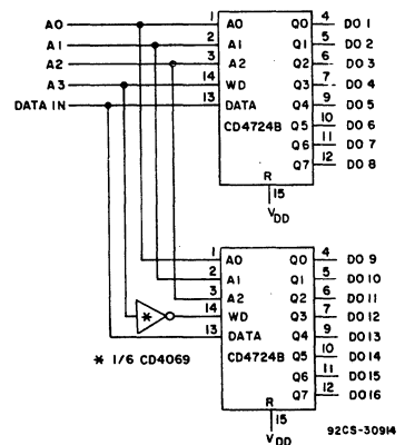
Fig. 14—1 of 16 decoder/demultiplexer.
