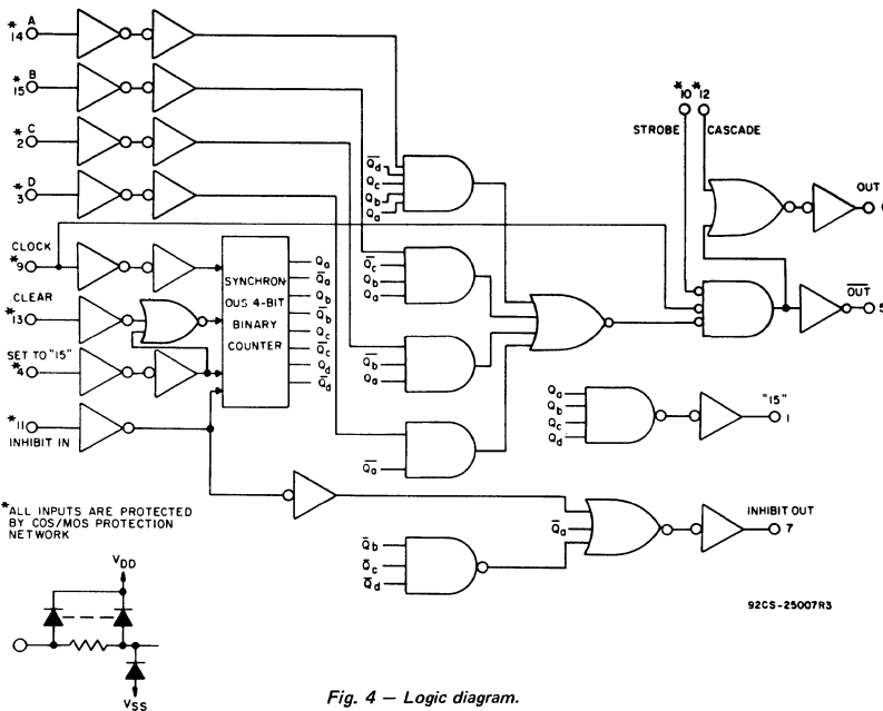
Fig. 4 - Logic diagram.
