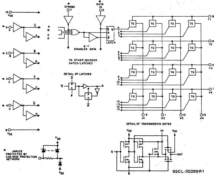
Fig. 6— Schematic diagram.
