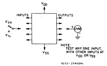
Fig. 15 – Input voltage.
