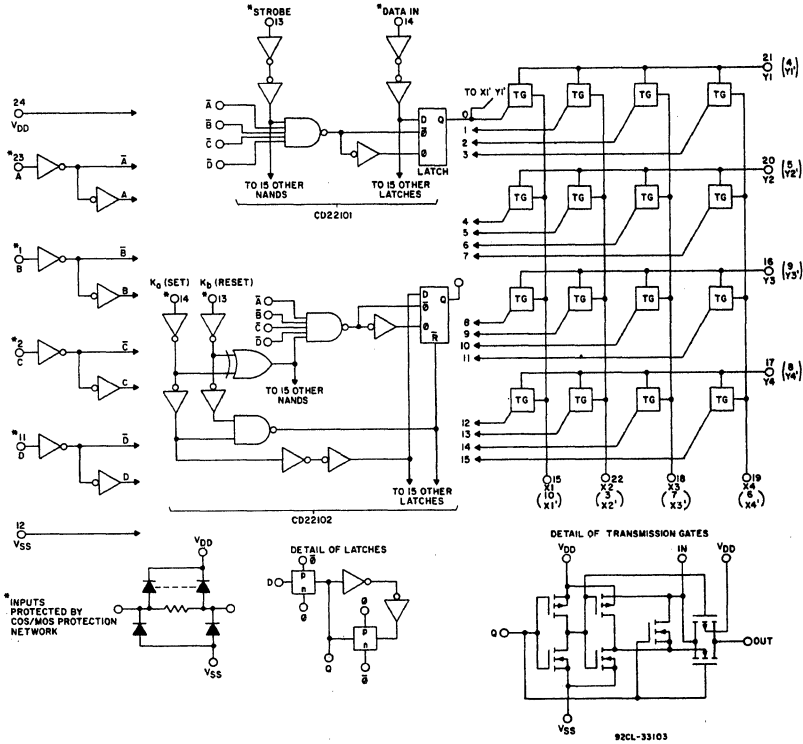
Fig. 2 - Logic diagram.
