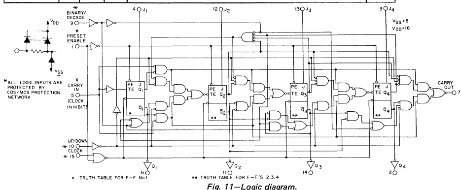
Fig. 11—Logic diagram.
