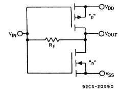
Fig. 5— COS/MOS amplifier.
