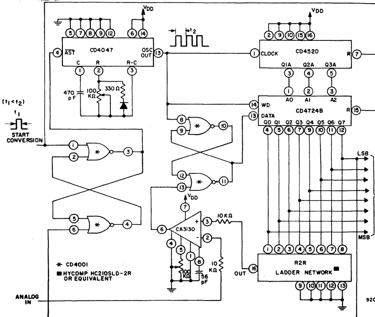
Fig. 5—A/D converter
