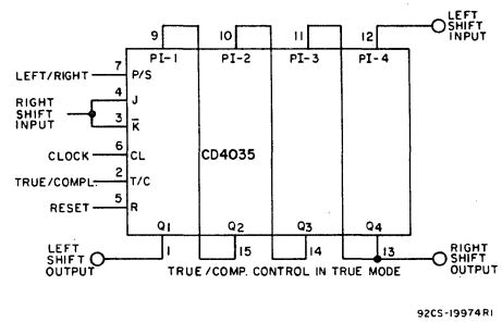
Fig. 14 - Shift left/shift right register.
