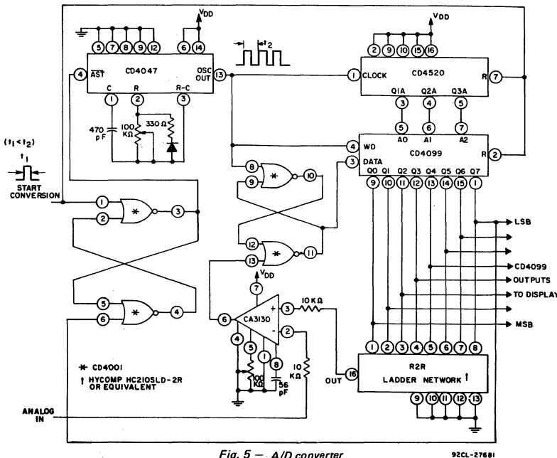
Fig. 5 - A/D converter
